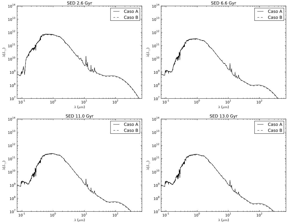
Figura 4.12: SEDs calculada para uma galáxia de 1 \times 10^{11} M_{\odot} para os casos A ( (\delta_{cond}^{II}(A), \delta_{cond}^{II}(A), \delta_{cond}^I(A)) = (1.0, 0.7, 0.7) ) e B ( (\delta_{cond}^{II}(C), \delta_{cond}^{II}(C), \delta_{cond}^I(C)) = (1.0, 0.5, 0.5) ) e (\delta_{cond}^{II}(Si), \delta_{cond}^{II}(Si), \delta_{cond}^I(Si)) = (1.0, 0.8, 0.8) ) de produção de poeira nos tempos 2.6 (superior esquerdo), 6.6 (superior direito), 11.0 (inferior esquerdo) e 13.0 Gano (inferior direito). As linhas tracejadas indicam o caso B e a contínua o A.
